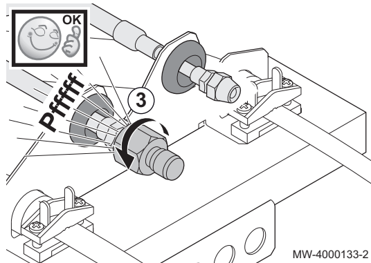
Fig.34 Dévisser les écrous
