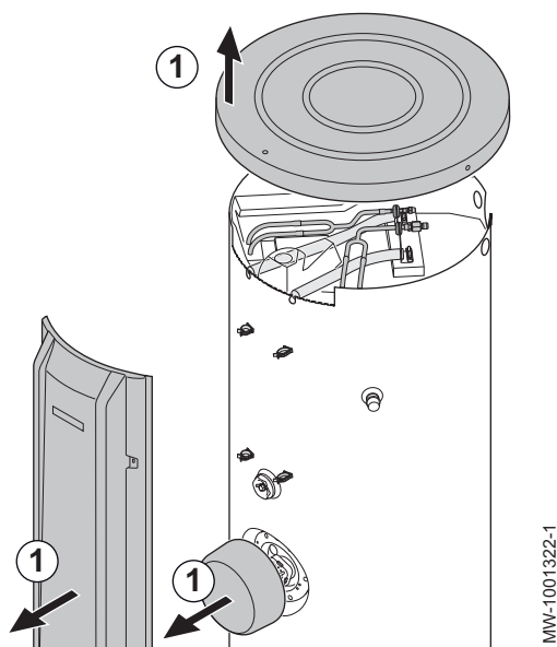
Fig.54 Passage des câbles
