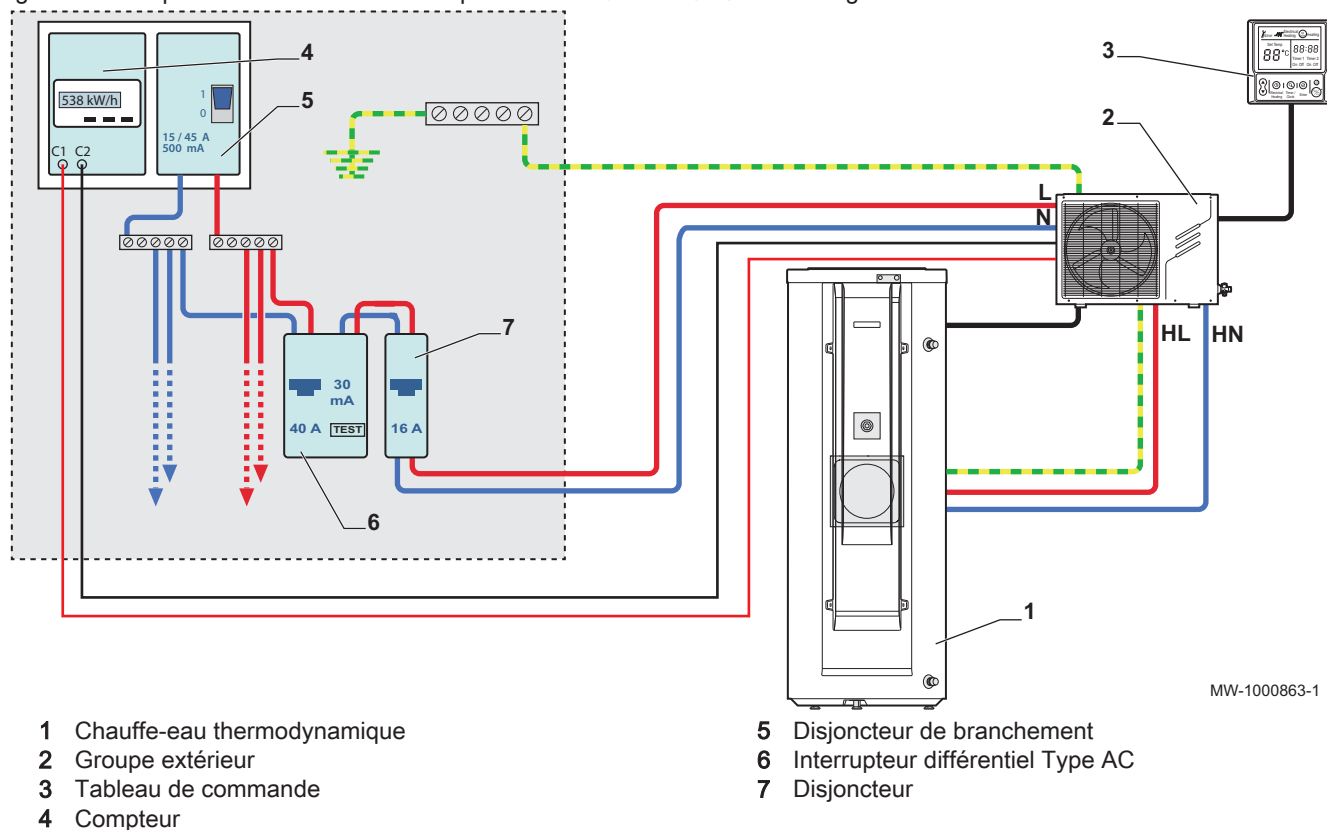
Fig.51 Exemple de raccordement électrique en mode OPT.BACKUP – Montage 2
