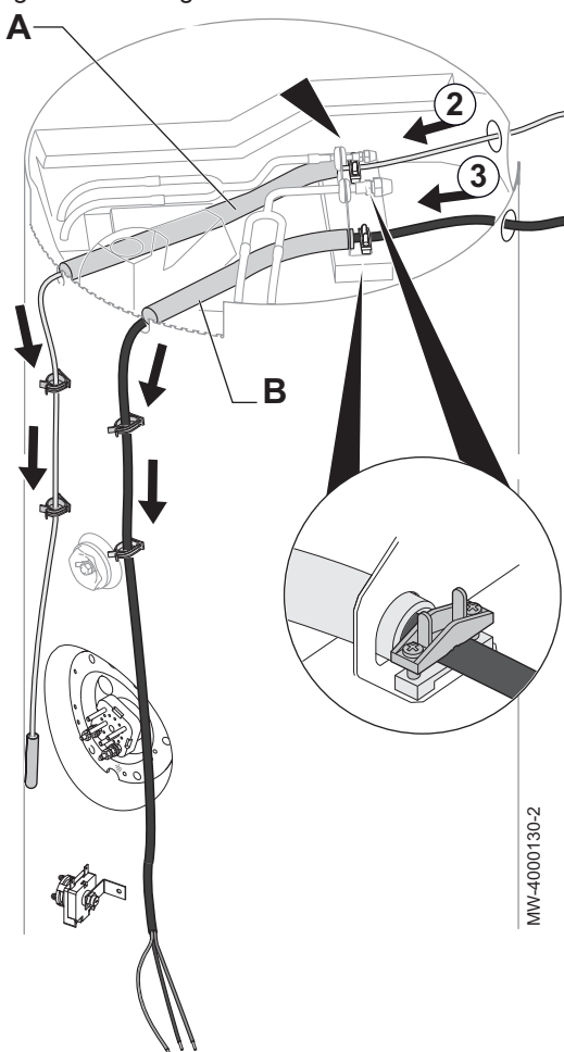
Fig.54 Passage des câbles
