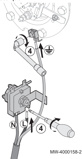
Fig.56 Mise en place de la sonde
