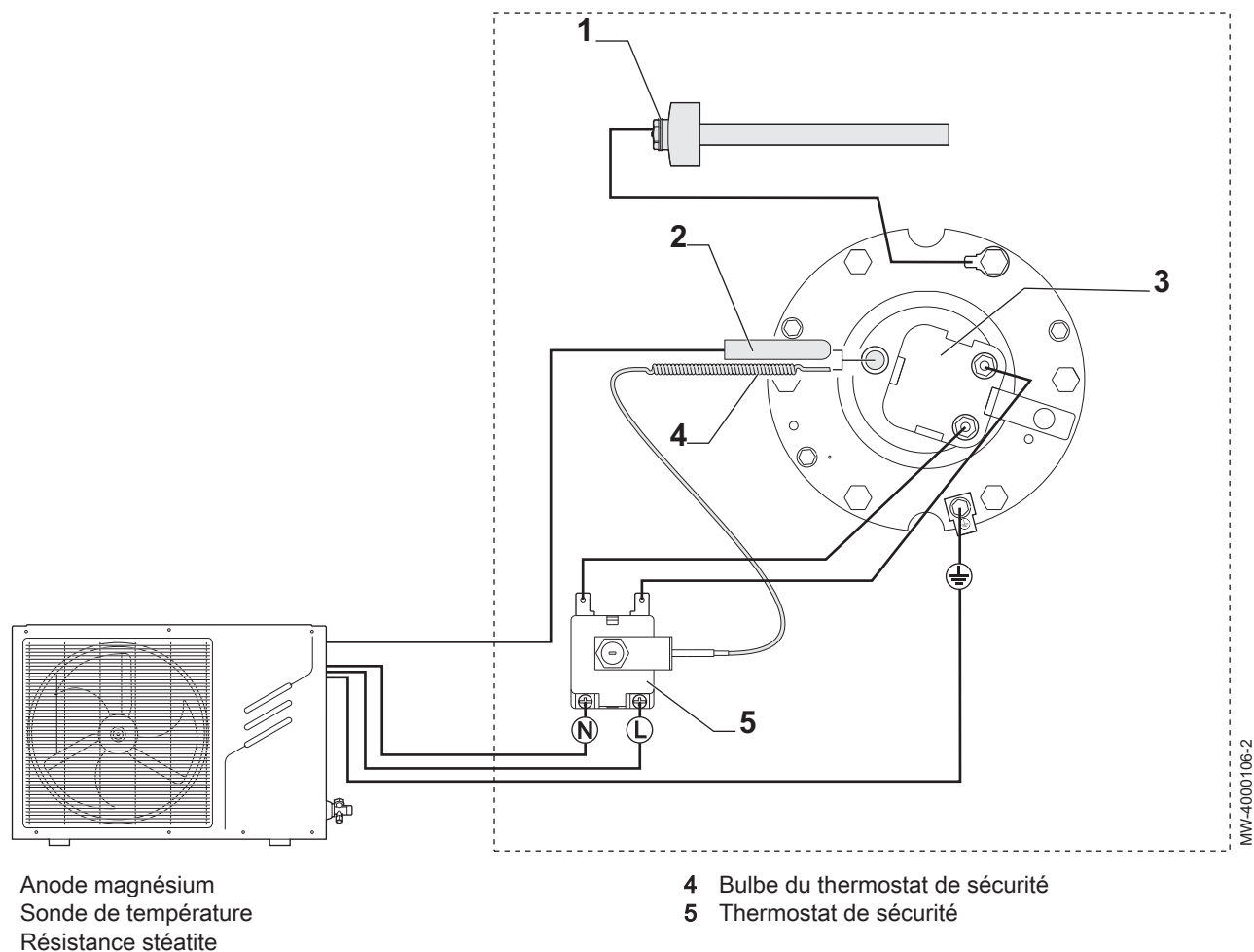
Fig.5 Schéma électrique
