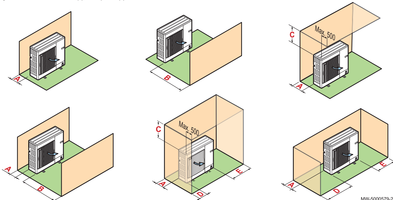
Fig.19 Distances de l'appareil par rapport au mur
