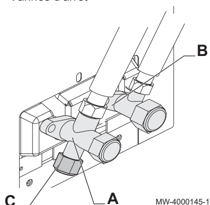
Fig.44 Vannes d'arrêt
