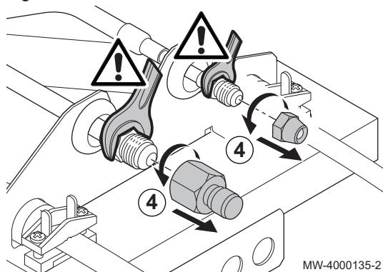
Fig.35 Mise au rebut des opercules
