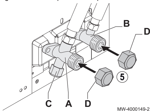
Fig.48 Mise en place des capuchons
