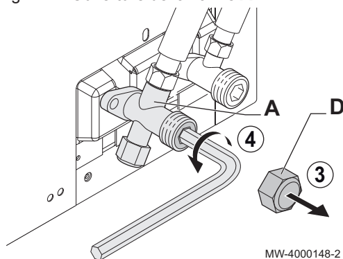
Fig.47 Ouverture de la vanne A
