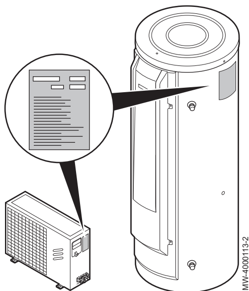
Fig.13 Emplacement des plaquettes signalétiques
