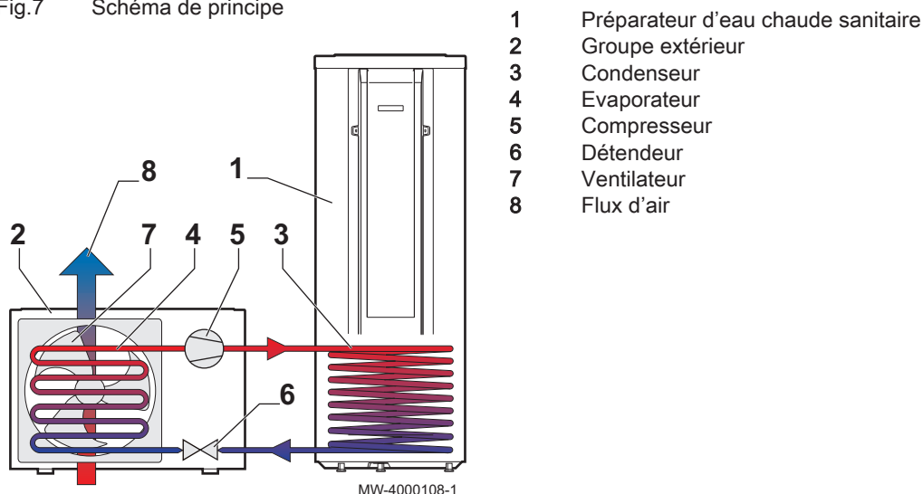
Fig.7 Schéma de principe
