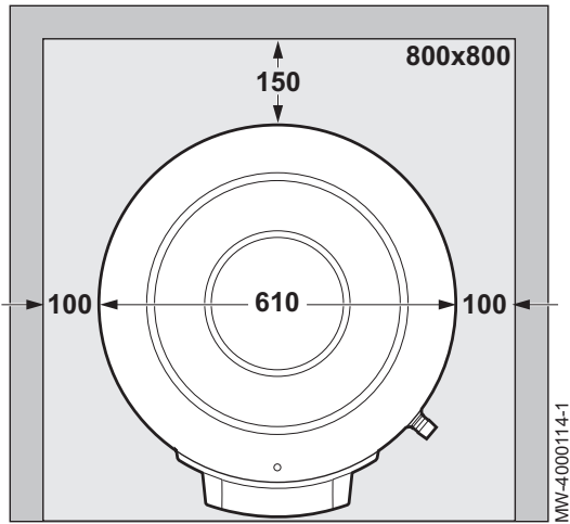
Fig.15 Emplacement à prévoir pour le préparateur d'eau chaude sanitaire
