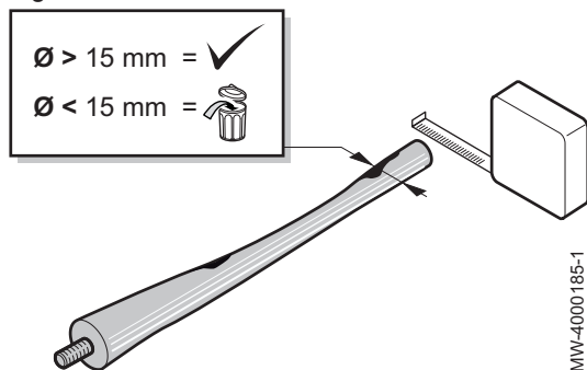
Fig.69 Contrôle de l'anode
