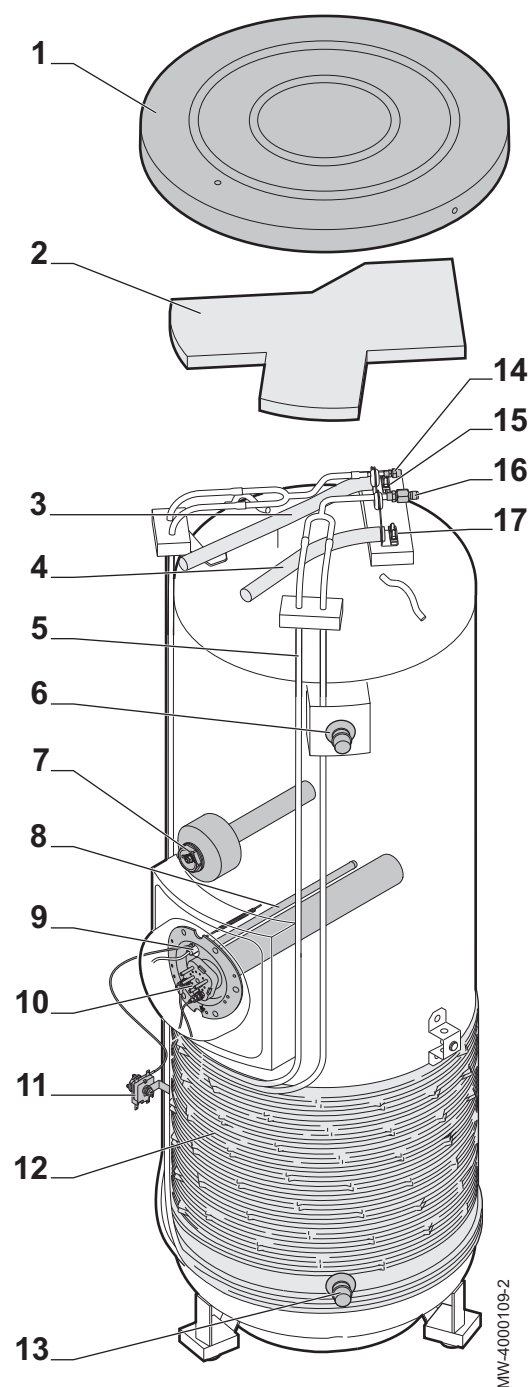
Fig.9 Principaux composants
