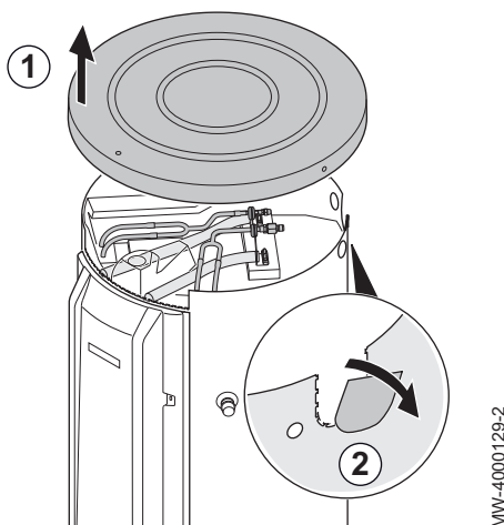
Fig.32 Découpe pour liaisons frigorifiques
