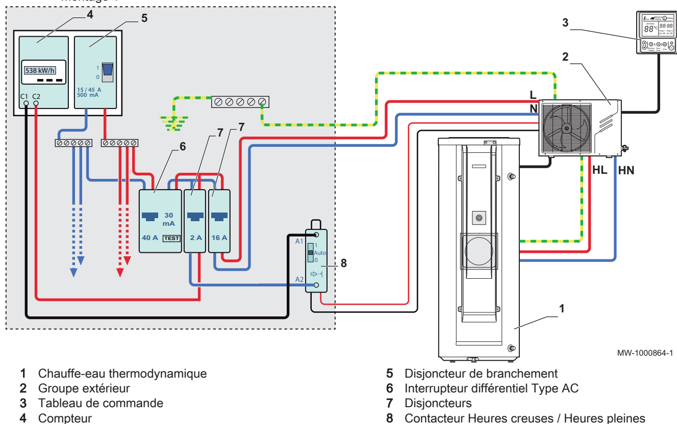
Fig.50 Exemple de raccordement électrique en mode OPT.BACKUP avec câbles HEURES CREUSES / HEURES PLEINES – Montage 1
