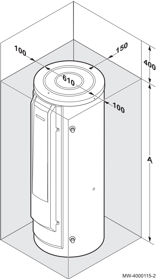
Fig.15 Emplacement à prévoir pour le préparateur d'eau chaude sanitaire
