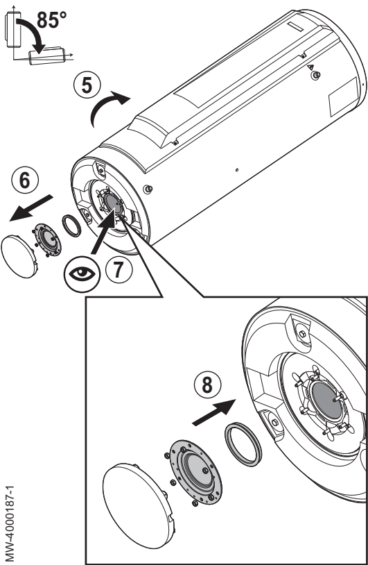
Fig.71 Accès à la trappe de visite inférieure
