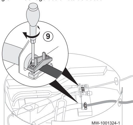
Fig.57 Serrage des arrêts de traction
