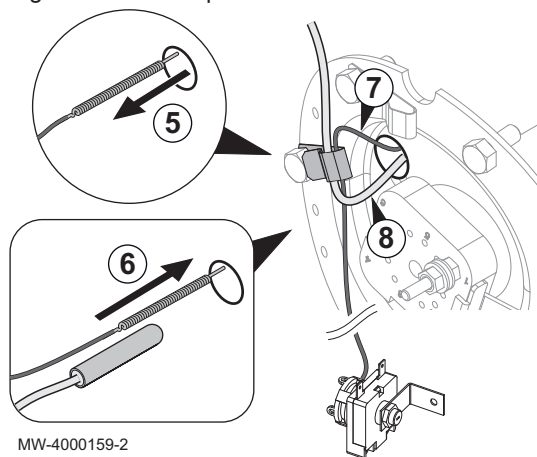
Fig.57 Serrage des arrêts de traction
